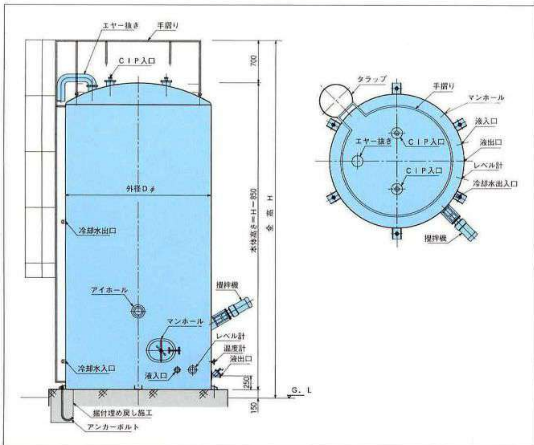
STS型標準寸法表
