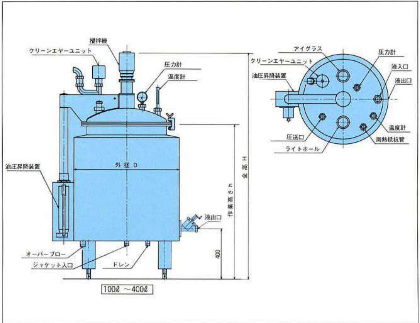
VTC型標準寸法表
