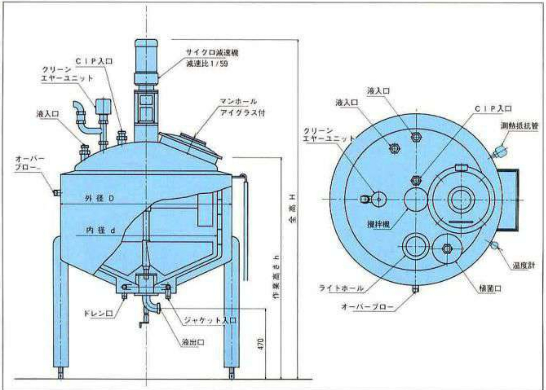
KTE型標準寸法表
